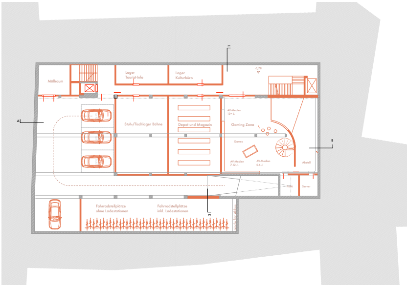
2. Untergeschoss 200
