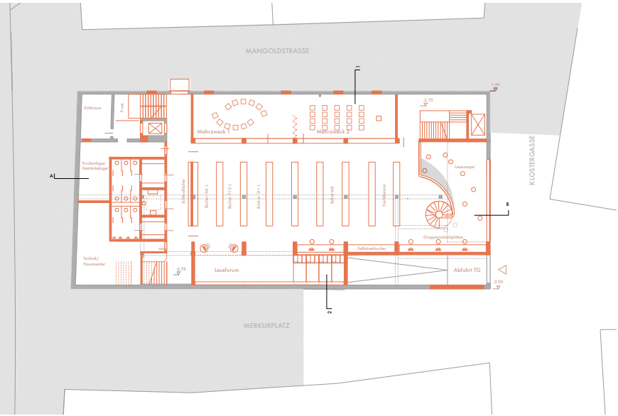
1. Untergeschoss 200
