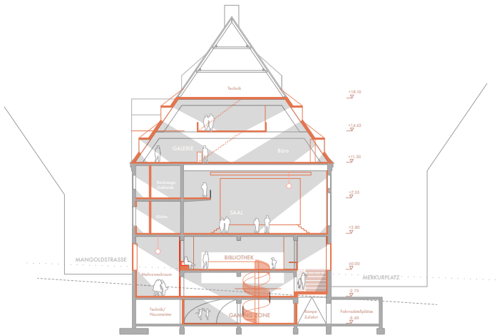
Schnitt 1-2 200
