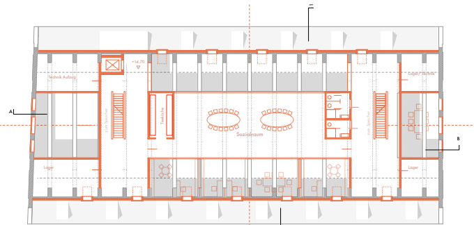
2. Dachgeschoss 200
