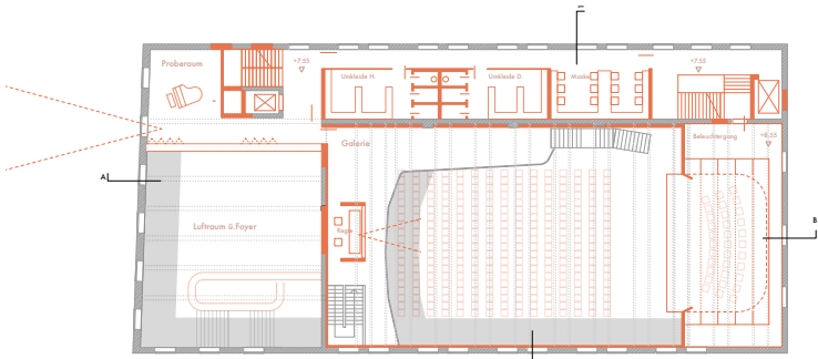
2. Obergeschoss 200
