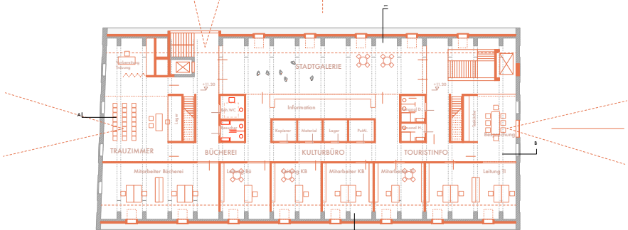
1. Dachgeschoss 200
