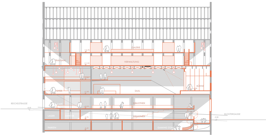
Schnitt A-B 200
