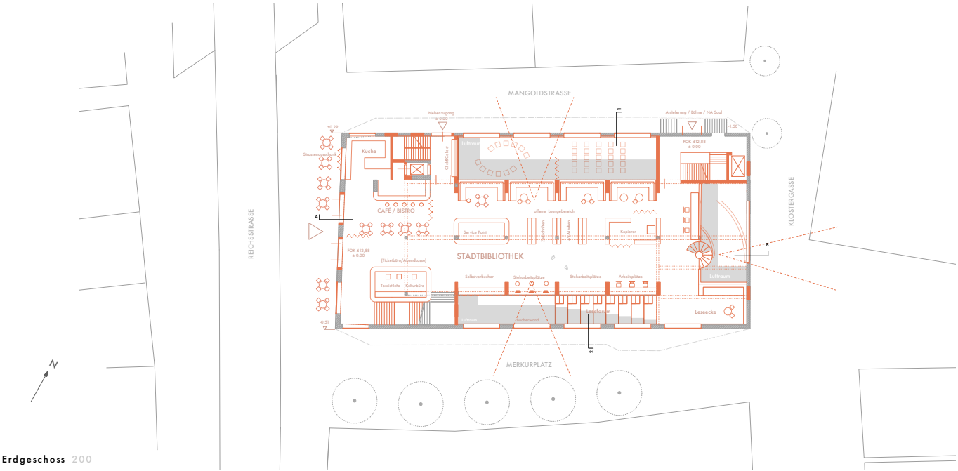
Erdgeschoss 200
