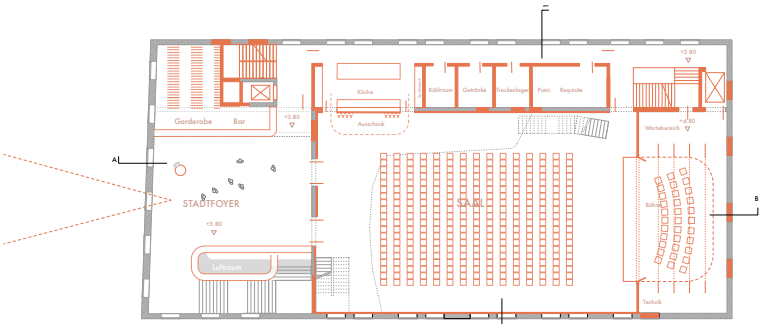
1. Obergeschoss 200
