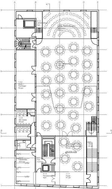
GRUNDRISS 1.OG 1:200 - BANKETTESTUHLUNG
