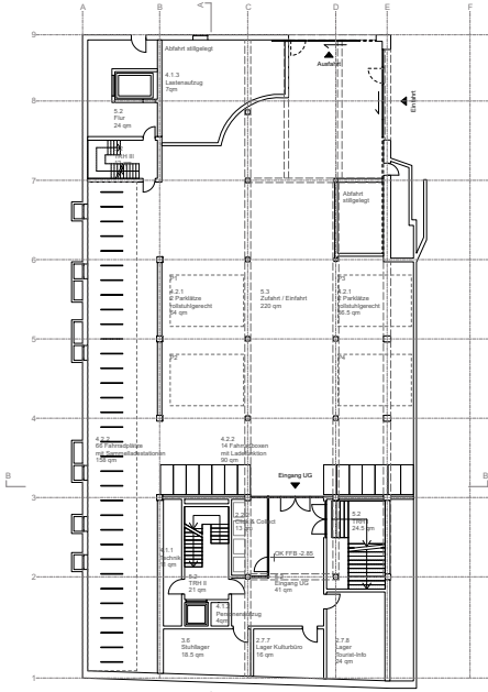
GRUNDRISS 1.UG 1:200
