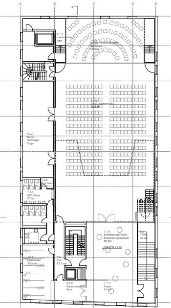
GRUNDRISS 1.OG 1:200 - REIHENBESTUHLUNG
