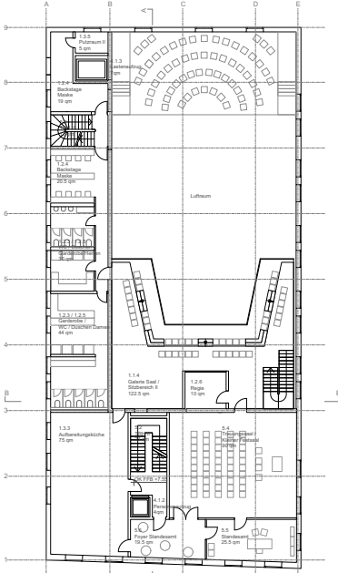
GRUNDRISS 2.OG 1:200 - REIHENBESTUHLUNG
