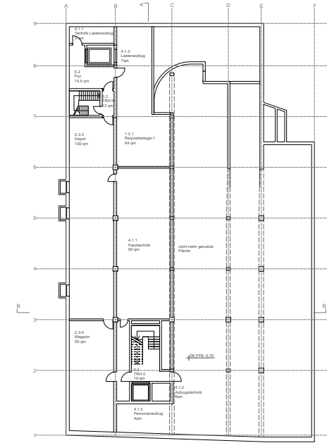
GRUNDRISS 2.UG 1:200
