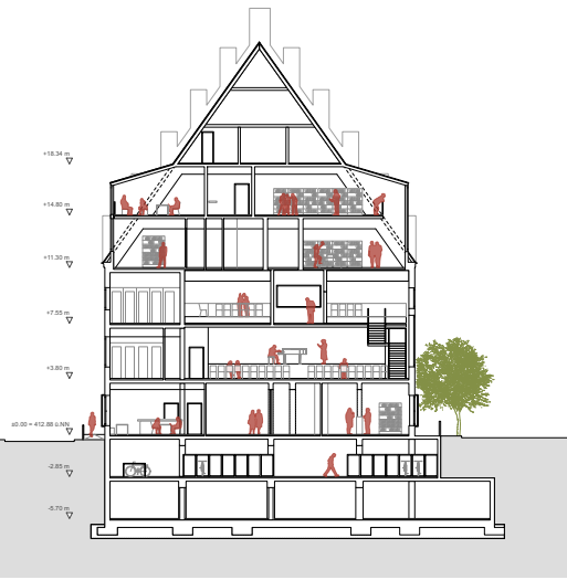
SNITT B-B 1:200
