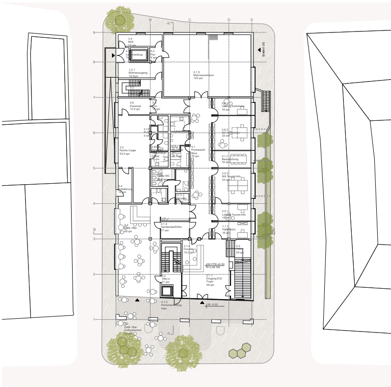
GRUNDRISS EG 1:200
