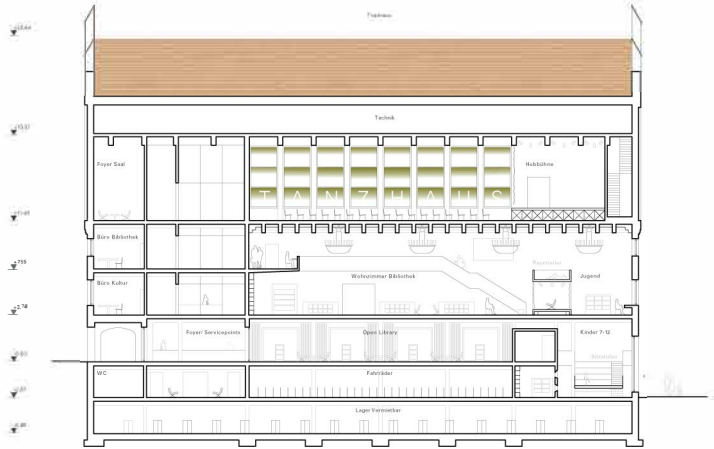
Längsschnitt B-B M 1:200
