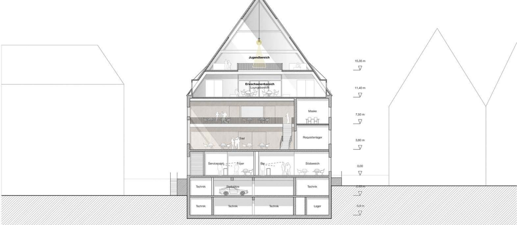
SCHNITT BB 1:200
