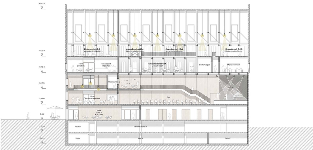
SCHNITT AA 1:200
